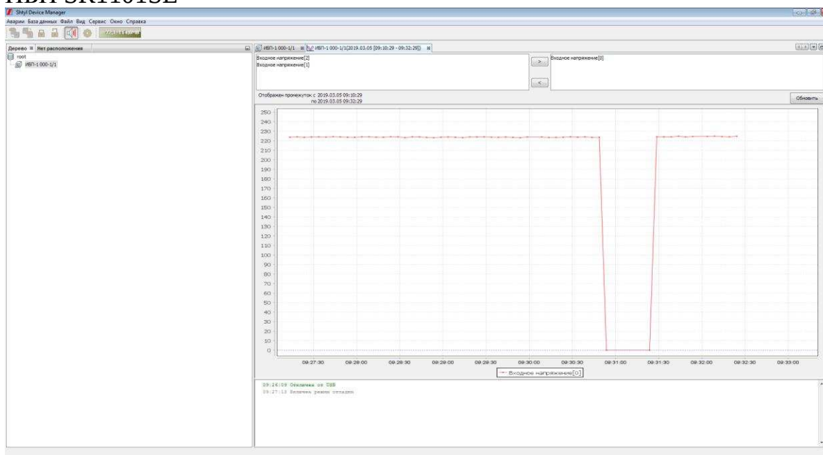
Рисунок 2.16 - Окно программы ShtylDeviceManager с отображением графика входного напряжения
