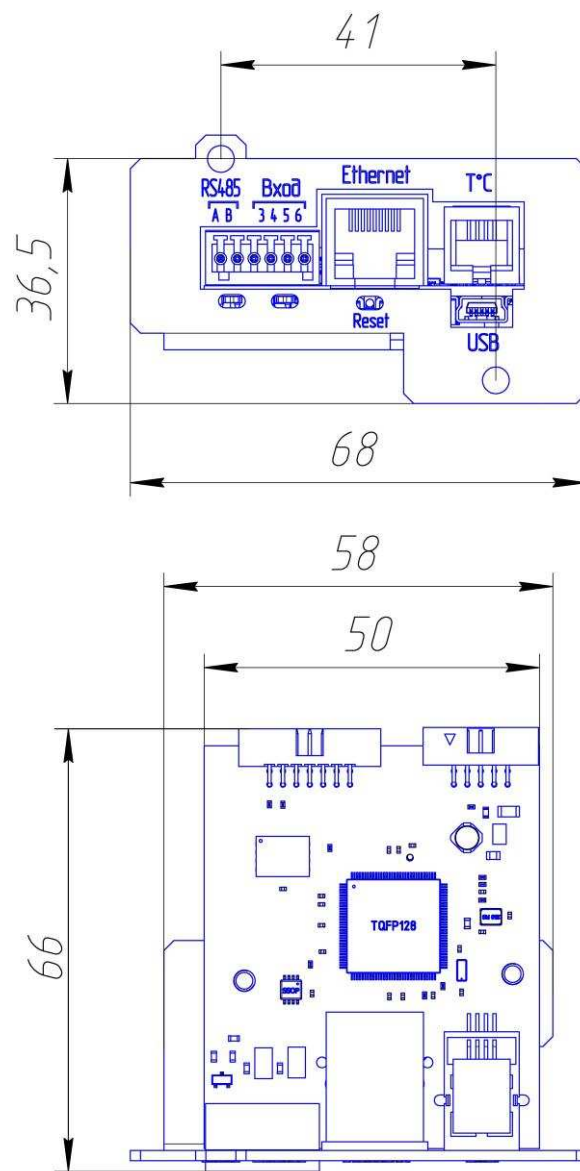
Рисунок 1.2 – Габаритные размеры изделия
