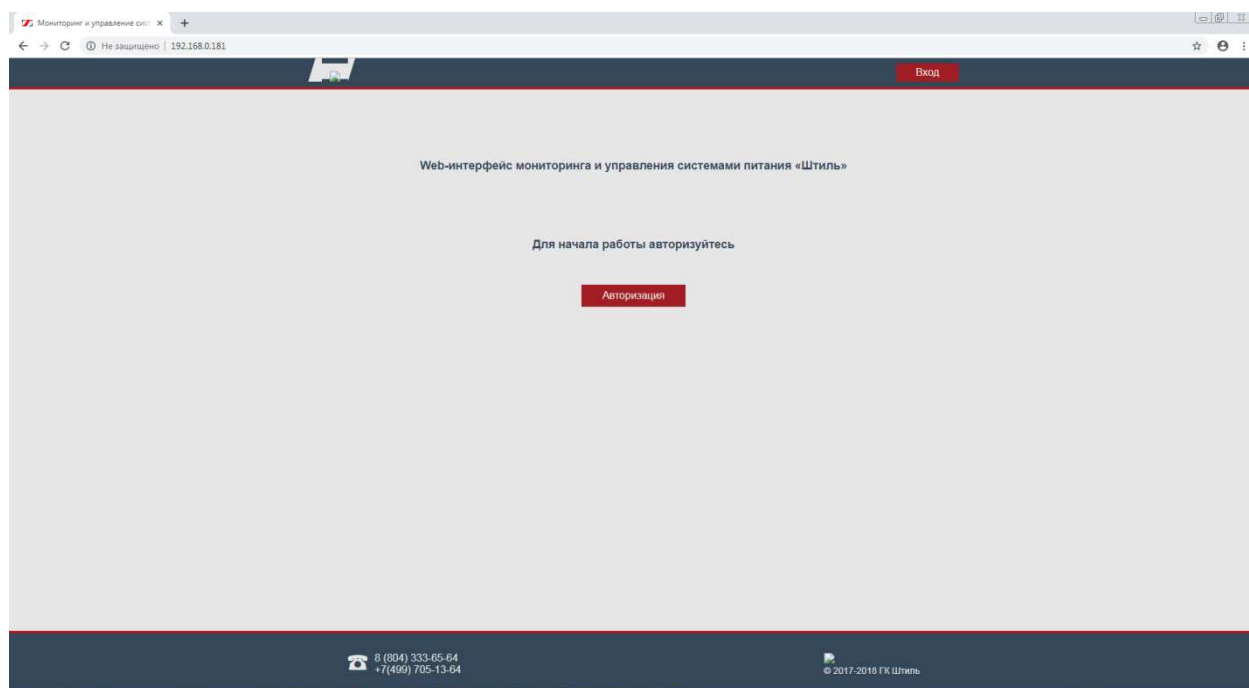
Рисунок 2.5 - Окно авторизации
