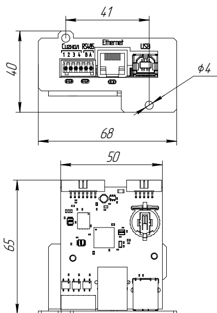
Рисунок 2. Габаритные размеры платы расширения интерфейсов ШТИЛЬ IC-SNMP/WEB
