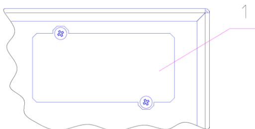
Рисунок 2.1 – Фрагмент тыльной стороны ИБП/стабилизатора с заглушкой интерфейсной платы
