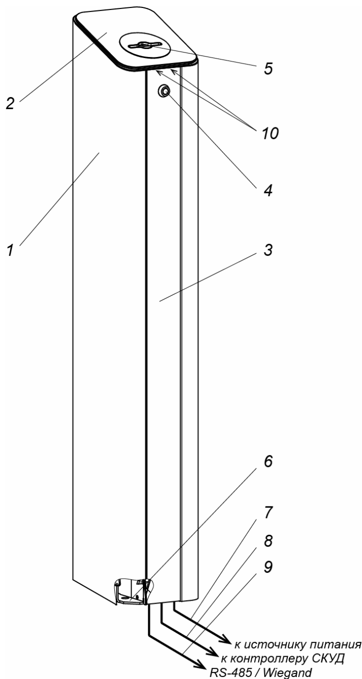
Рисунок 2. Устройство картоприемника:
