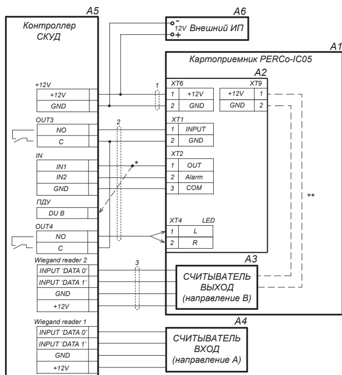
Схема подключения контроллеру СКУД по интерфейсу Wiegand
