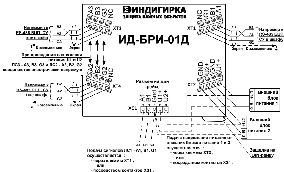
Рис. Подключение ИД-БРИ-01Д
