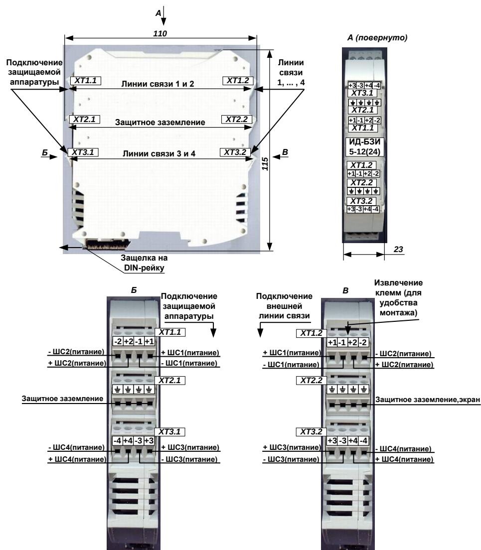
Рис. 2 Подключение, конструкция, размеры ИД-БЗИ-01Д
