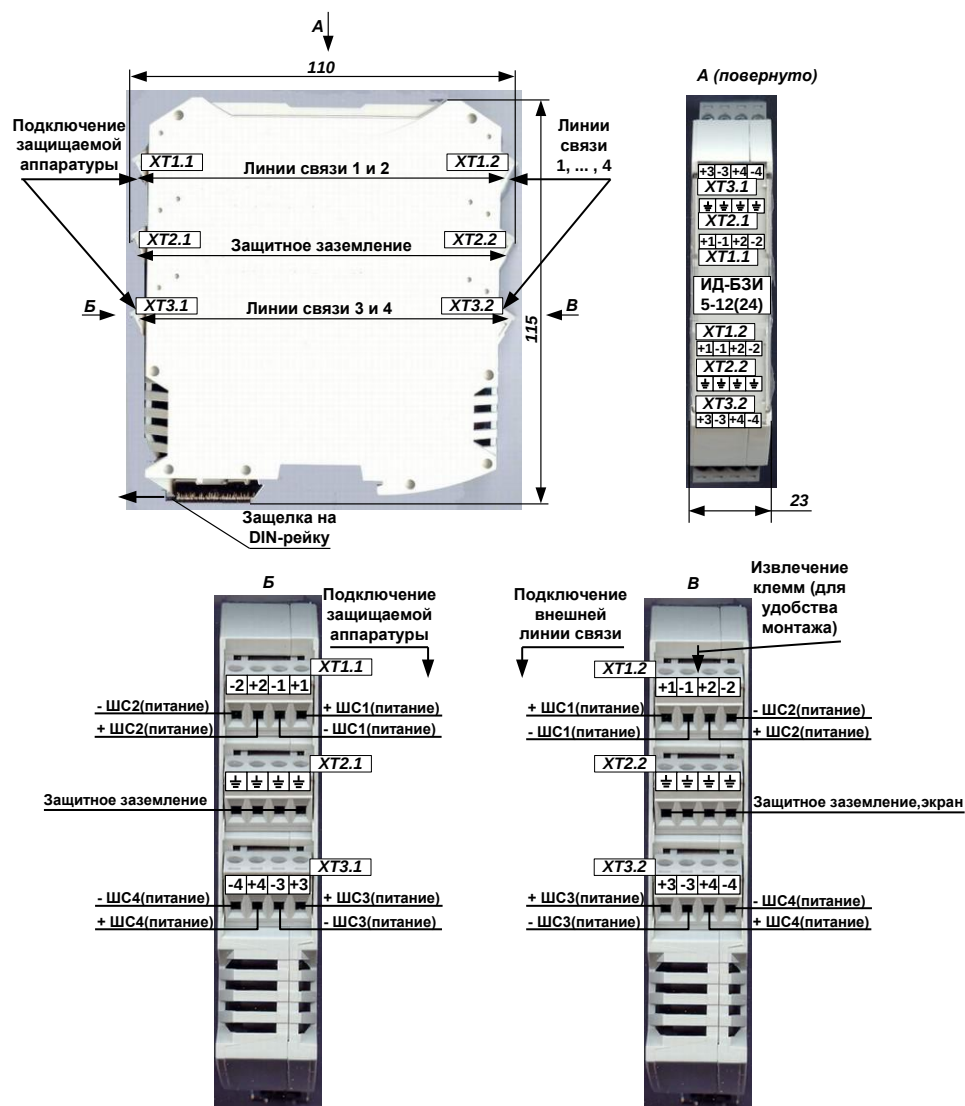
Рис. 2 Подключение, конструкция, размеры ИД-БЗИ-02Д
