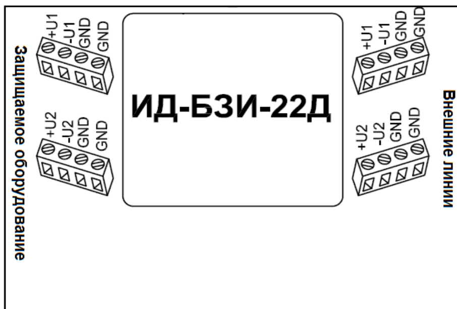
Рис. 2 Подключение ИД-БЗИ-22Д
