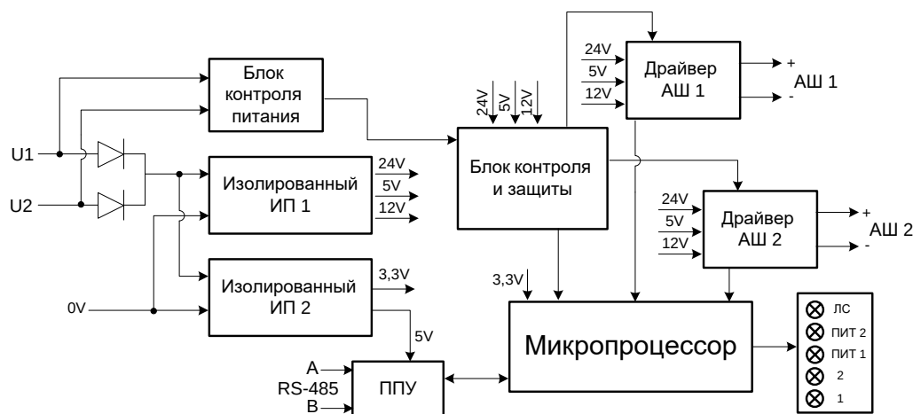
Рис. 2 Блок-схема ИД-КАУ-04Д
