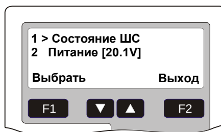
Рис. 6 Проверка монитора питания ПСФ
