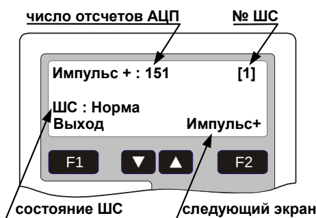
Рис. 7 Окно состояния ШС («Все»)
