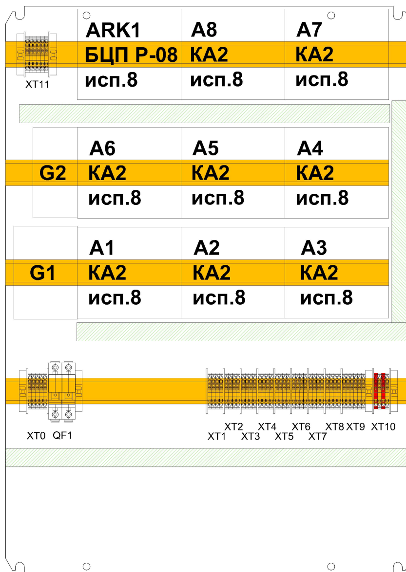
Рис. 3 Расположение оборудования на монтажной панели
