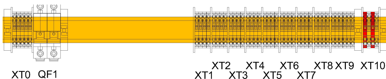
Рис. 4 Расположение клемм для подключения внешнего оборудования
