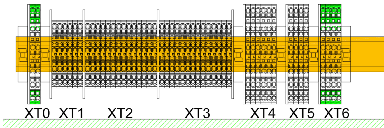
Рис. 2 Расположение клемм для подключения внешнего оборудования
