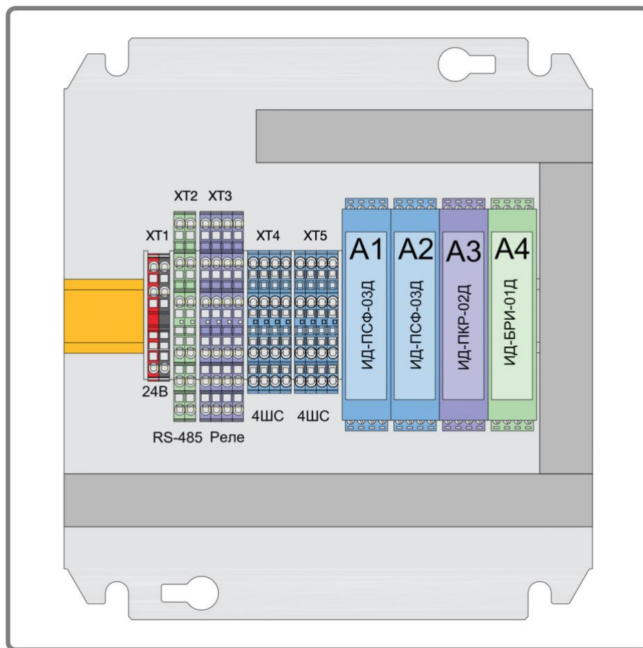
Рис. 2 Расположение оборудования на монтажной панели
