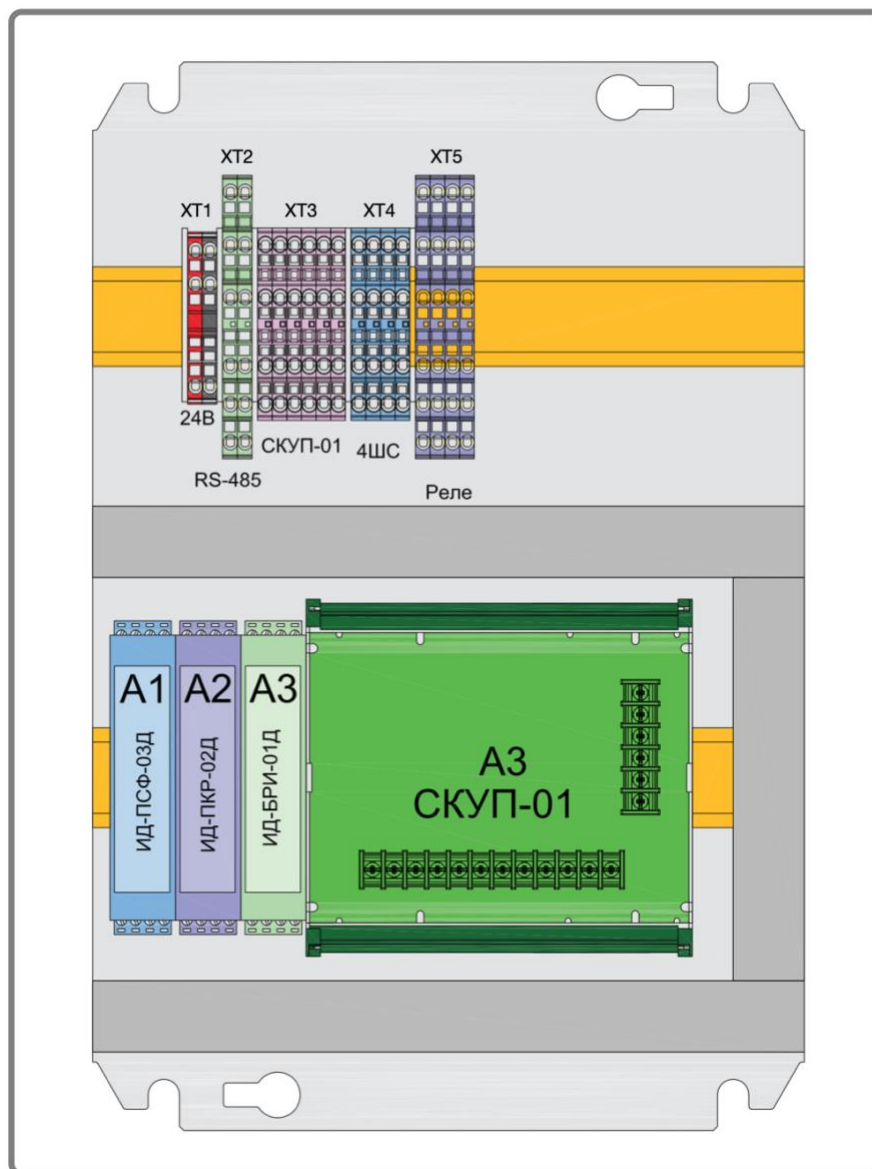
Рис. 2 Расположение оборудования на монтажной панели
