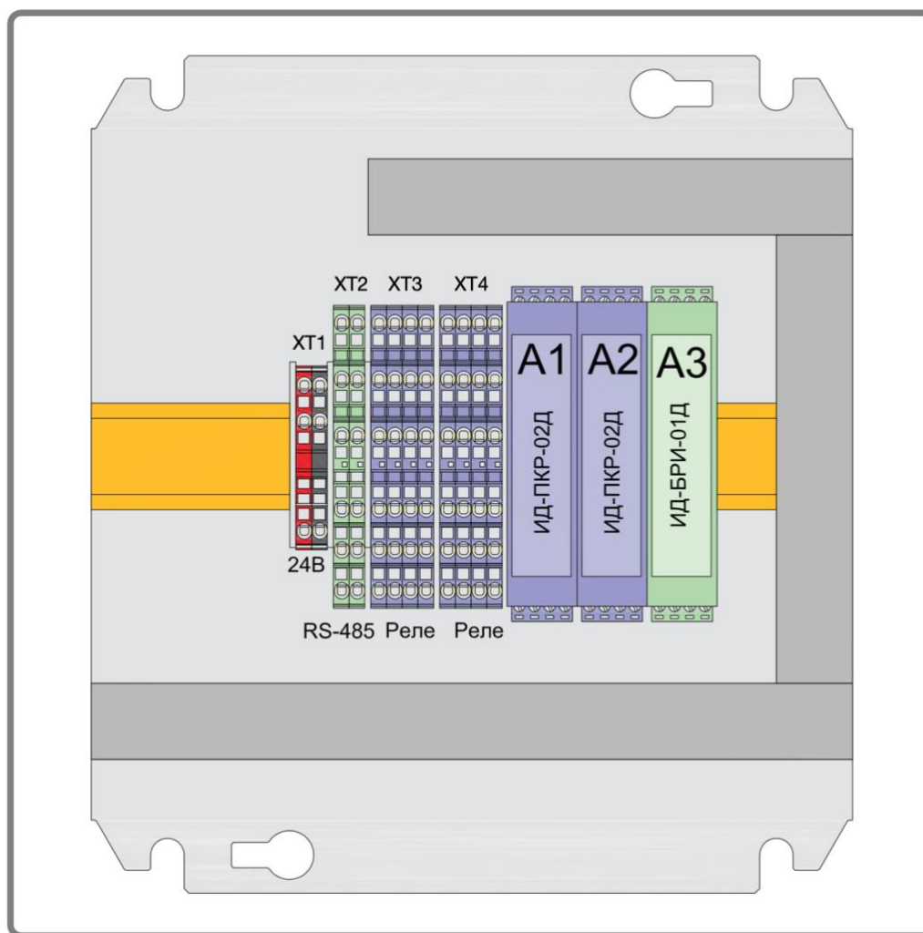
Рис. 2 Расположение оборудования на монтажной панели
