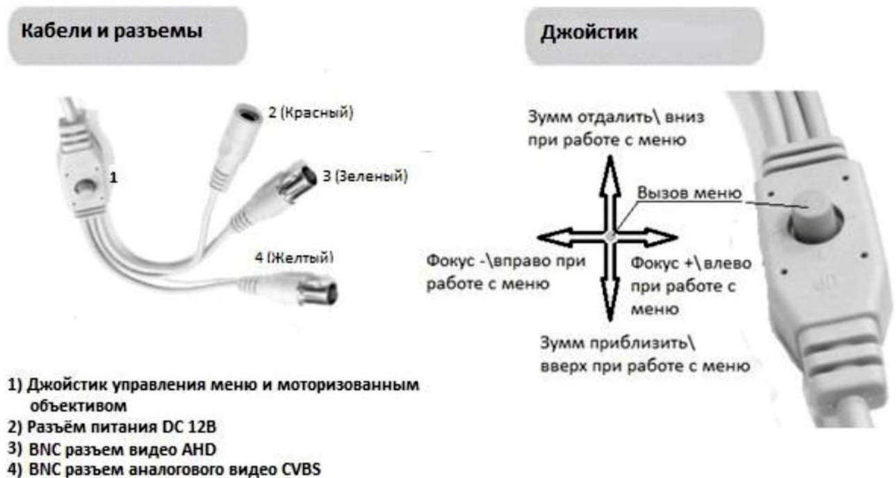
Рис. 3 Подключение и установка.
