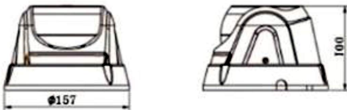
Рис. 2 Габаритные размеры.
