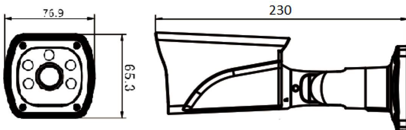
Рис. 2 Габаритные размеры.
