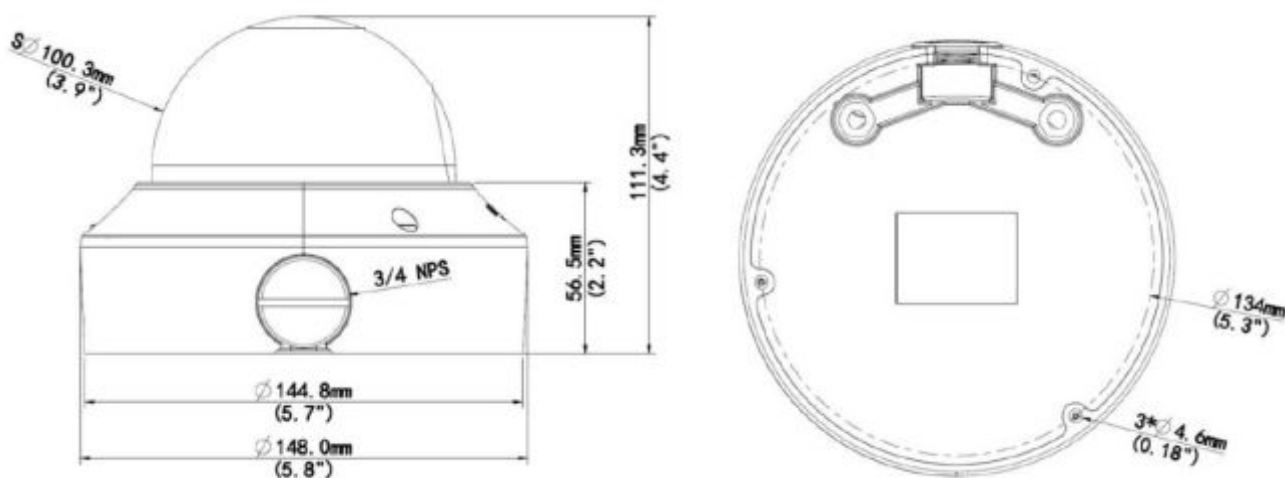
Рис. 2 Габаритные и присоединительные размеры.
