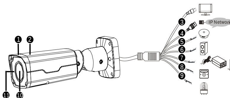
Рис. 4 Конструкция и разъемы подключения видеокамеры с кронштейном
