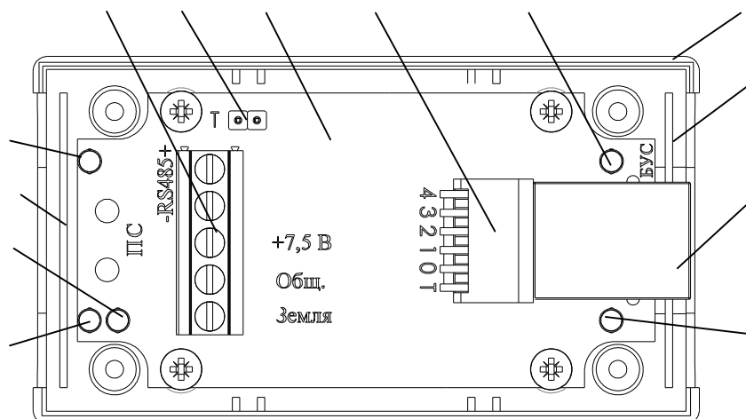
Рисунок 6.1. Вид на БСПС со снятой крышкой. 1 – винтовой клеммник для присоединения к ПС, 2 – переключатель включения терминатора для интерфейса ПС, 3 – печатная плата, 4 – переключатель задания адреса и управления терминатором шины СОУЭ, 5 – индикатор обмена данными с БУС, 6 – корпус, 7, 12 – заглушки, 8 – соединитель для присоединения к БУС, 9 – индикатор ошибки работы с БУС, 10 – индикатор ошибки работы с ПС, 11 – индикатор питания, 13 – индикатор обмена данными с ПС.
