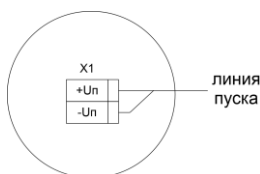
Рисунок 2 – Схема внешних подключений ИИУ-07-Ех
