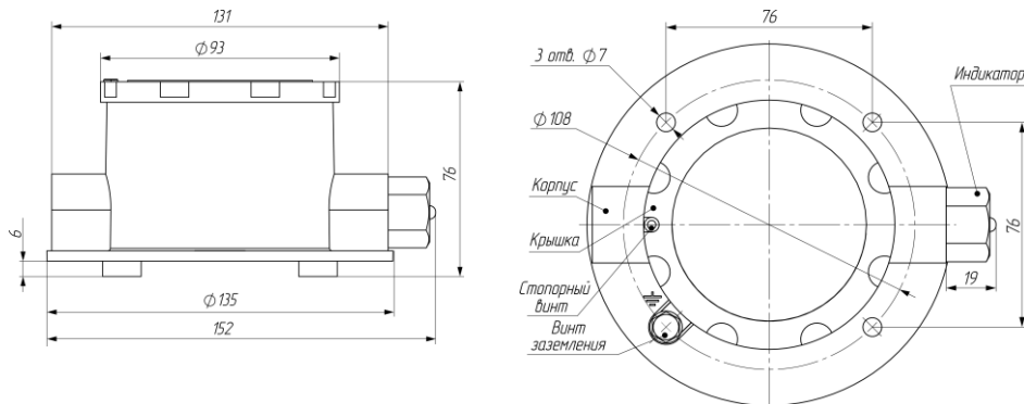
Рисунок 1 – Габаритные и установочные размеры ИИУ-07-Ех
