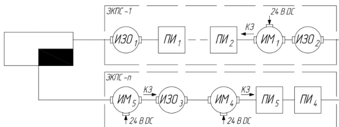
Рисунок 9 – Схема структурная включения ИМ-Ех-П в кольцевую двухпроводную АЛС для имитации обрыва и КЗ между ЗКПС
