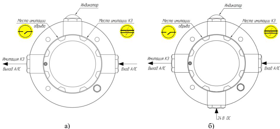
Рисунок 1 – Внешний вид ИМ-Ех-П с обозначением мест имитации:
