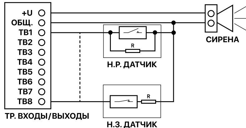
Рис.2 Тревожные входы/выходы видеодомофона
