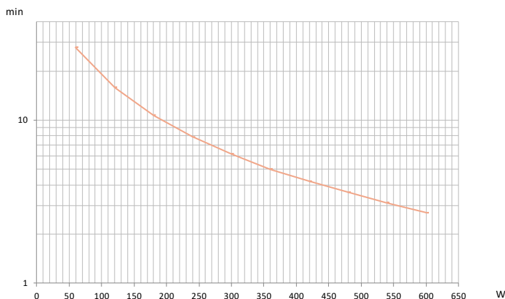
Figura 6. Grafico della durata della batteria INFOPDU1000PL / INFOPDU1000LCD
