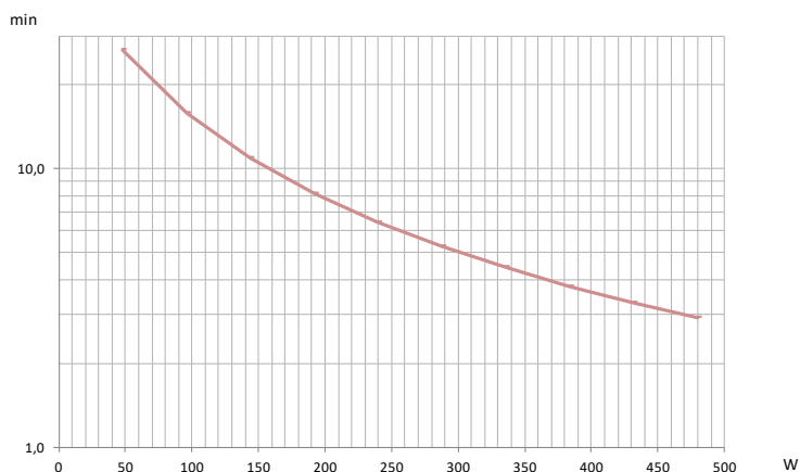
Figura 5. Grafico della durata della batteria INFOPDU800 / INFOPDU800PL / INFOPDU800LCD
