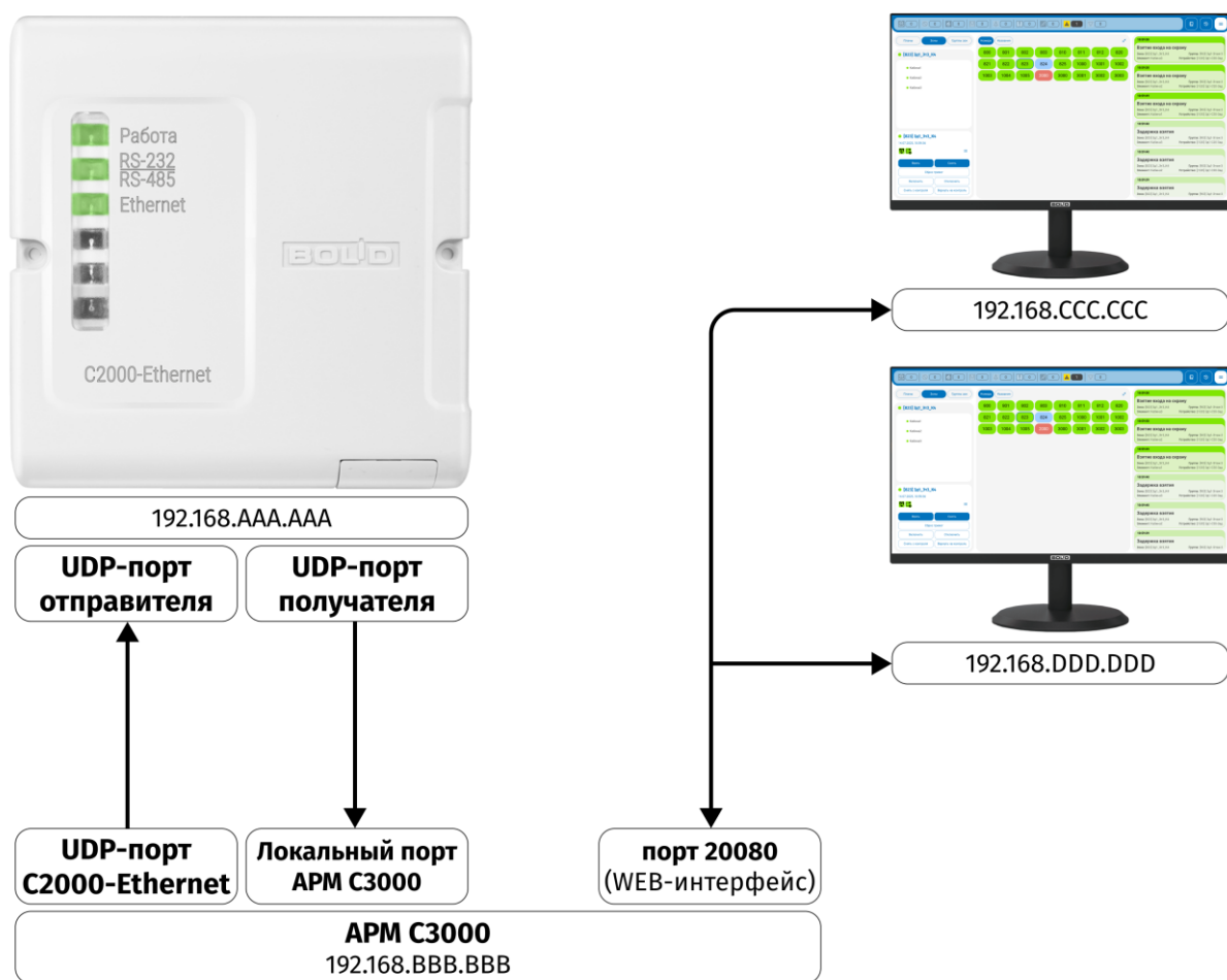
Рисунок 97. Общая схема соответствия параметров конфигураций «C2000-Ethernet» и АРМ «С3000»
