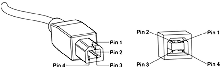
Рис. 8. Порт USB "папа" (слева), и "мама" (справа)
