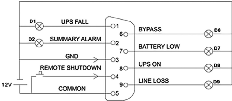
Figura 11. Stato UPS tramite connettore DB-9
