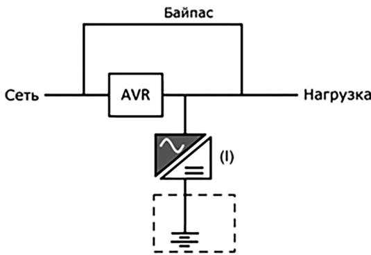
Рис. 1. Блок-схема
