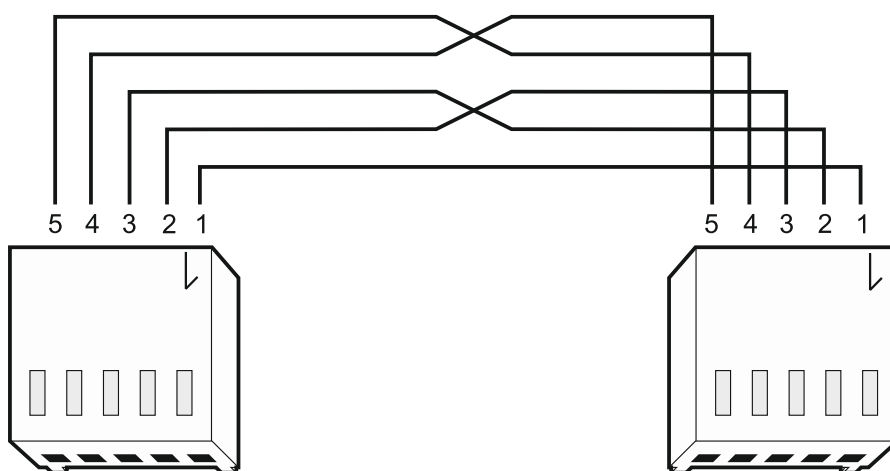
Рис. 6. Схема кабеля, предназначенного для подключения порта RS-232 модуля INT-GSM к прибору INTEGRA с разъемом PIN5.
