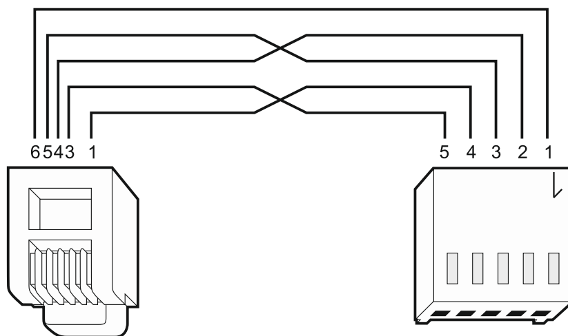
Рис. 5. Схема кабеля, предназначенного для соединения порта RS-232 модуля INT-GSM и прибора INTEGRA / INTEGRA Plus с разъемом типа RJ.
