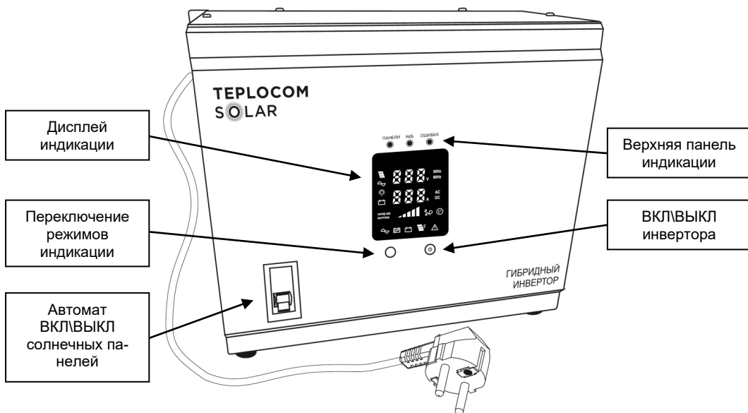
Рисунок 3 – Лицевая сторона инвертора Teplocom Solar 1500
