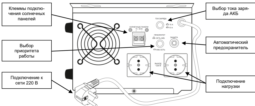
Рисунок 4 – Боковая сторона инвертора Teplocom Solar 1500
