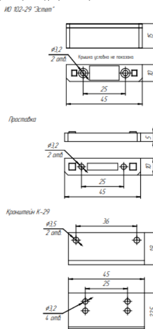
Рис.4 Габаритные и присоединительные размеры.
