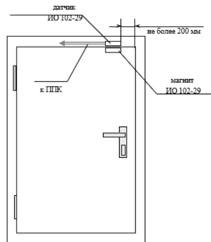
Рисунок 2. Пример установки извещателя для охраны дверного проема
