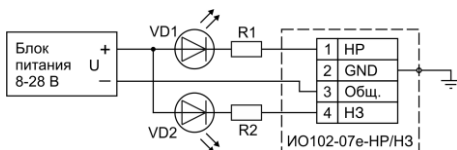
Рисунок 6. Расположение клемм и схемы внутренних соединений неадресных извещателей ИО102-07е
