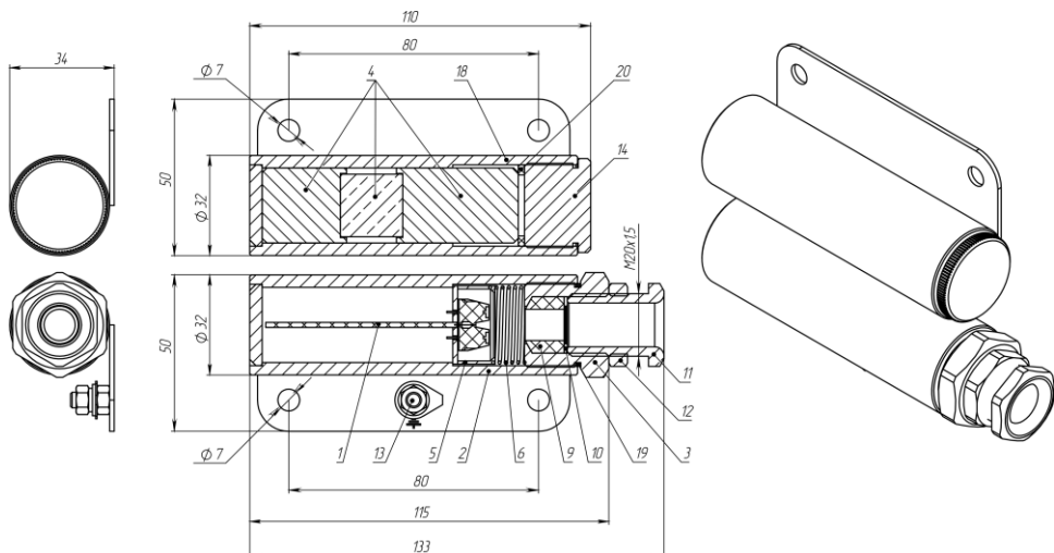
а) корпус из нержавеющей стали ИО102-07е-02П-Н
