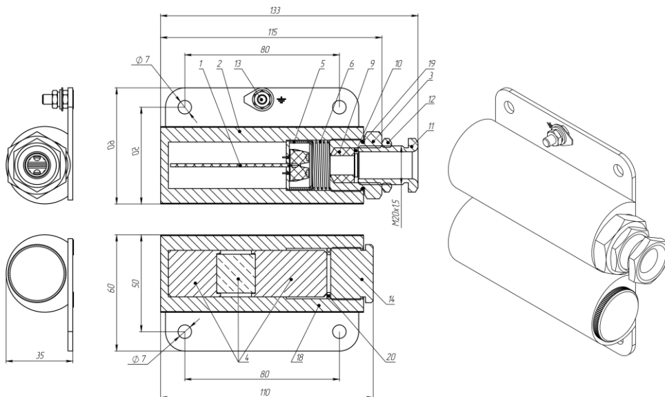
б) корпус из алюминиевого сплава ИО102-07е-02Л-А
