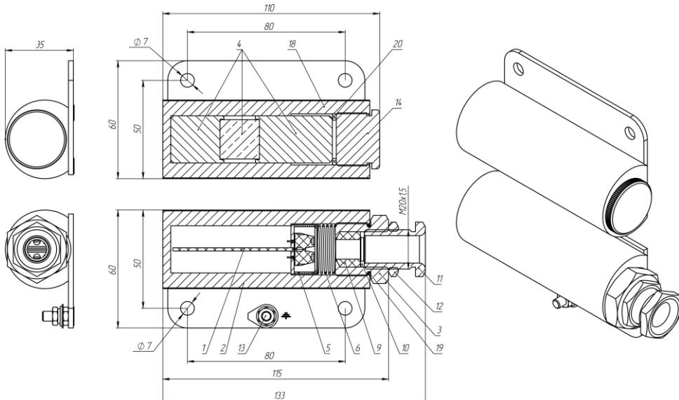
б) корпус из алюминиевого сплава ИО102-07е-02П-А
