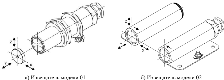
Рисунок 4 - Схема расположения и относительного перемещения блоков датчика и магнита извещателей ИО102-07ea
