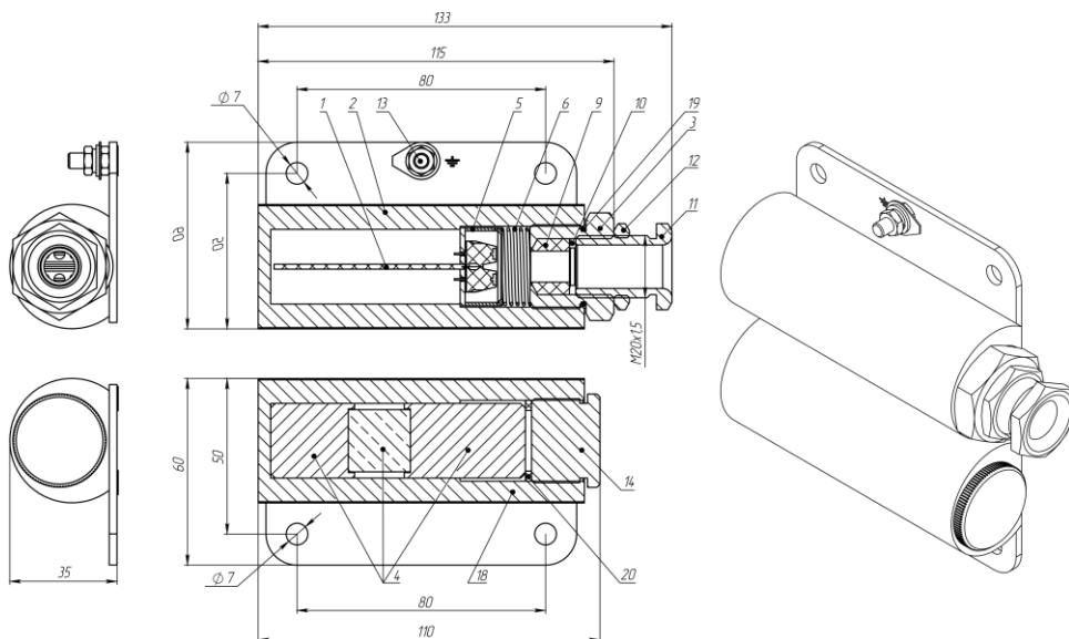
б) корпус из алюминиевого сплава ИО102-07еа-02Л-А
