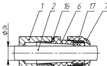
е) монтаж в кабельном вводе КВП12
