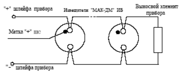
Рис. 2 Типовая схема включения извещателей в шлейфы сигнализации взрывозащищенных приемно-контрольных приборов
