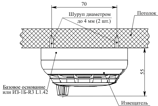
Рисунок А.1 – Установка извещателя на несущем потолке или каркасе подвесного потолка с базовыми основаниями W1.02, W1.03 или ИЗ-1Б-РЗ L1.42
