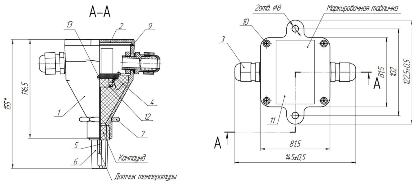
Рис. А3. Конструкция и габаритные размеры теплового извещателя: неадресные ИП 101 – 216.53 – А3 – ГРИФОН-Ехi-У, ИП 101 – 216.54 – С – ГРИФОН-Ехi-У, ИП 101 – 216.55 – D – ГРИФОН-Ехi-У.
