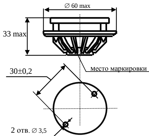
Габаритные и присоединительные размеры извещателя
