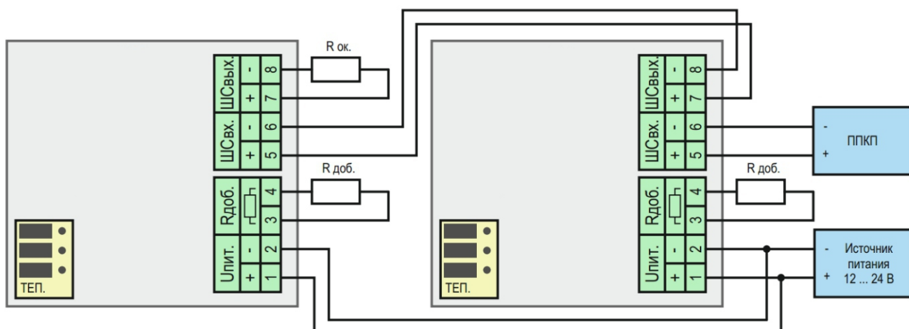
Схема подключения в ШС по последовательной схеме как извещателя с НЗ контактами (по принципу тепловых извещателей)
