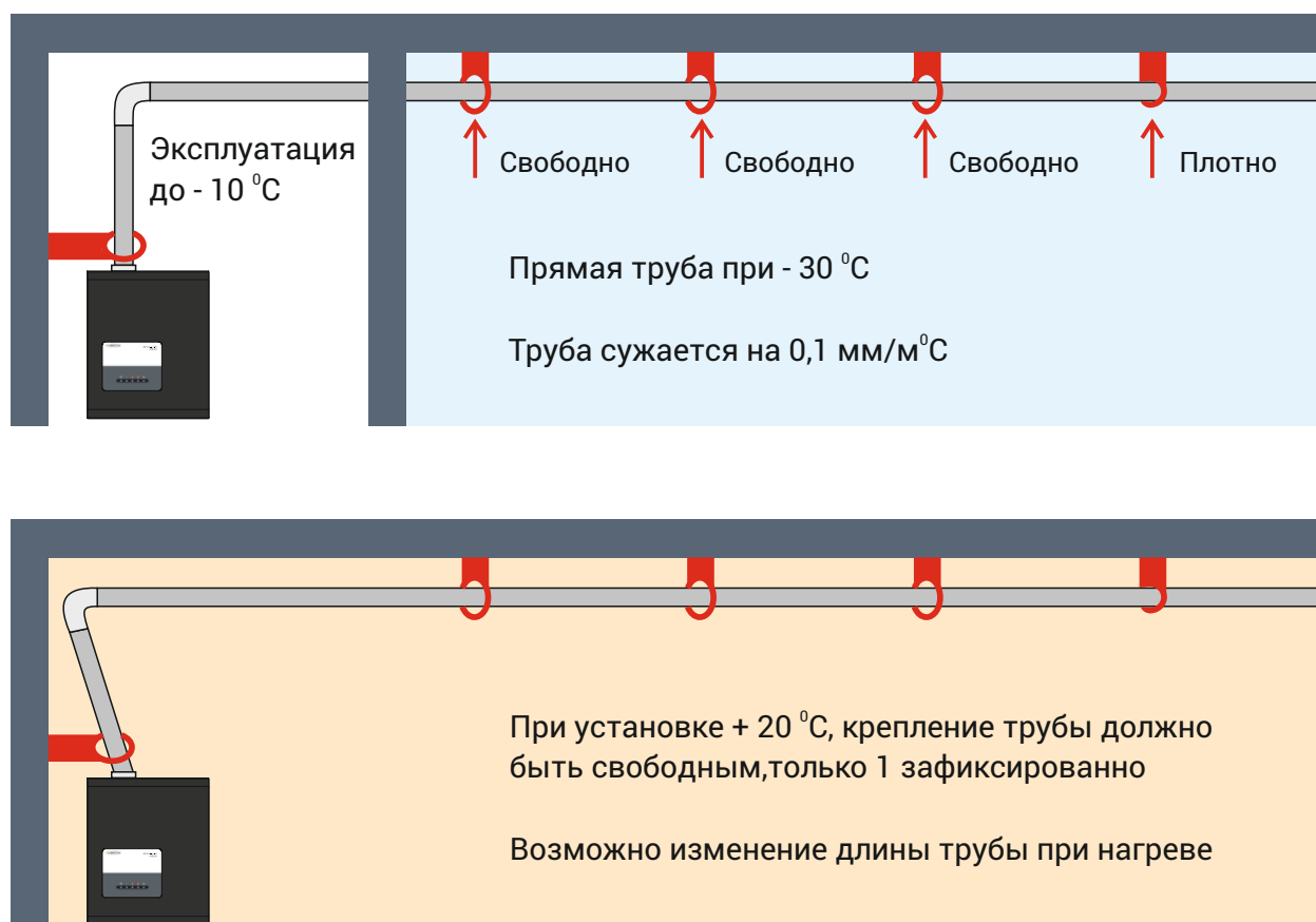
Рис. 5. Прокладка труб при отрицательных температурах
