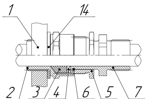
в) Прокладка кабеля в трубе с внешней резьбой г) Прокладка кабеля в металлорукаве
