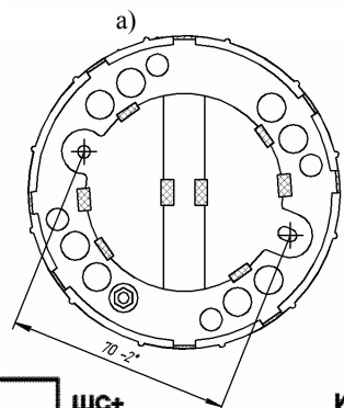
Рисунок 2. Вид на розетку с обратной стороны
