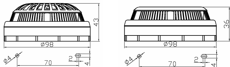
Рисунок 1. Габаритные и установочные размеры извещателей:
