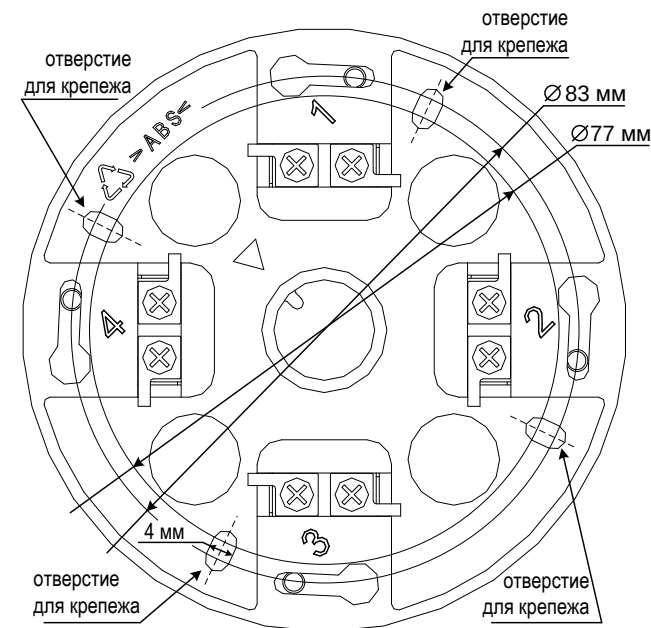
Рис.4 Базовое основание извещателя. Расположение отверстий для крепежа.
