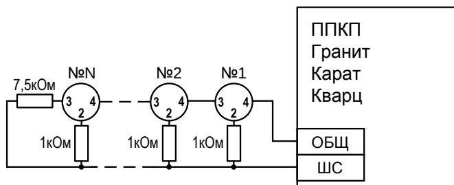
Рис.3 Схема подключения извещателей к ППКП «Гранит», «Карат» и «Кварц» производства ООО НПО «Сибирский Арсенал».
