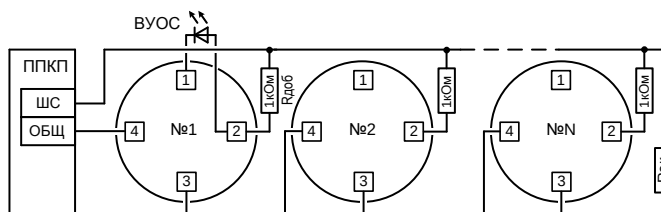
Рис.1 Типовая схема подключения извещателей к ППКП со знакопостоянным ШС. Величина резистора R_{ок} определяется в соответствии с техническим описанием ППКП. Добавочный резистор R_{доб} устанавливается – 1 кОм.
