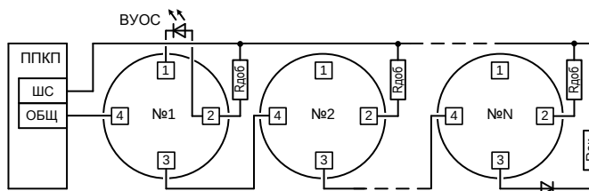
Рис.2 Типовая схема подключения извещателей к ППКП со знакопеременным ШС. Величина резисторов R_{ок} и R_{доб} определяется в соответствии с техническим описанием ППКП.
