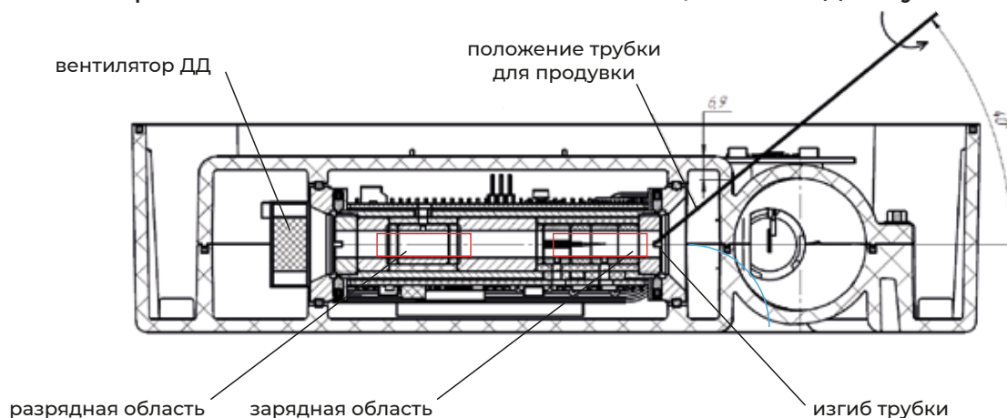
Рисунок 1 – Расположение трубки баллона для продувки датчика дыма
