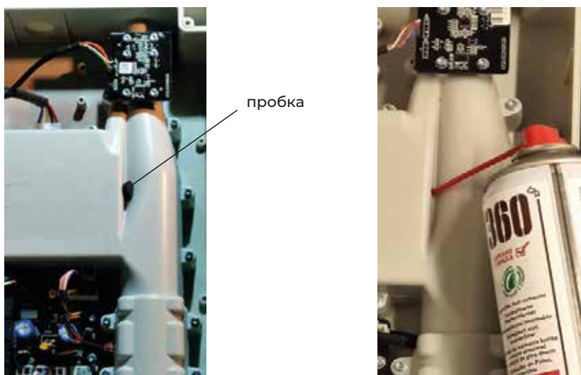
Рисунок 2 – Продувка трубки датчика дыма сжатым воздухом
