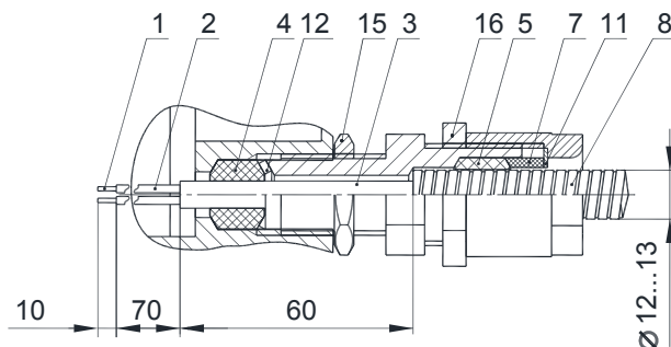
Рис. Б.2 Небронированный кабель в металлорукаве в внешнем диаметре 12..13мм в штупере ШБМ-Exd
