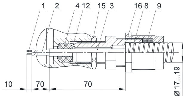
Рис. Б.3 Небронированный кабель в металлорукаве в внешнем диаметре 17..19мм в штупере ШБМ-Exd
