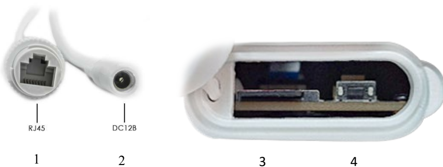
Рис. 1.2 Интерфейсы IP-камеры
