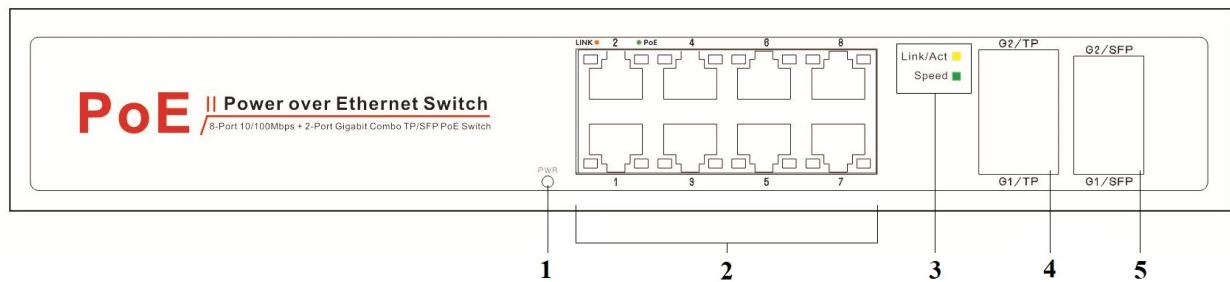
Рисунок 1 - Эскиз передней панели коммутатора.
