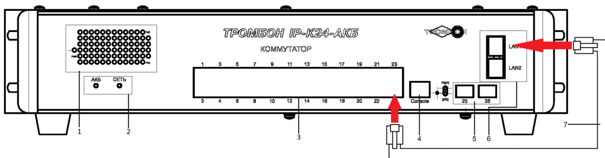
Рисунок 1 - Передняя панель коммутатора
