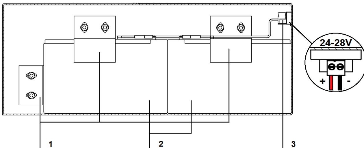
Рисунок 3 - Отсек установки аккумуляторных батарей
