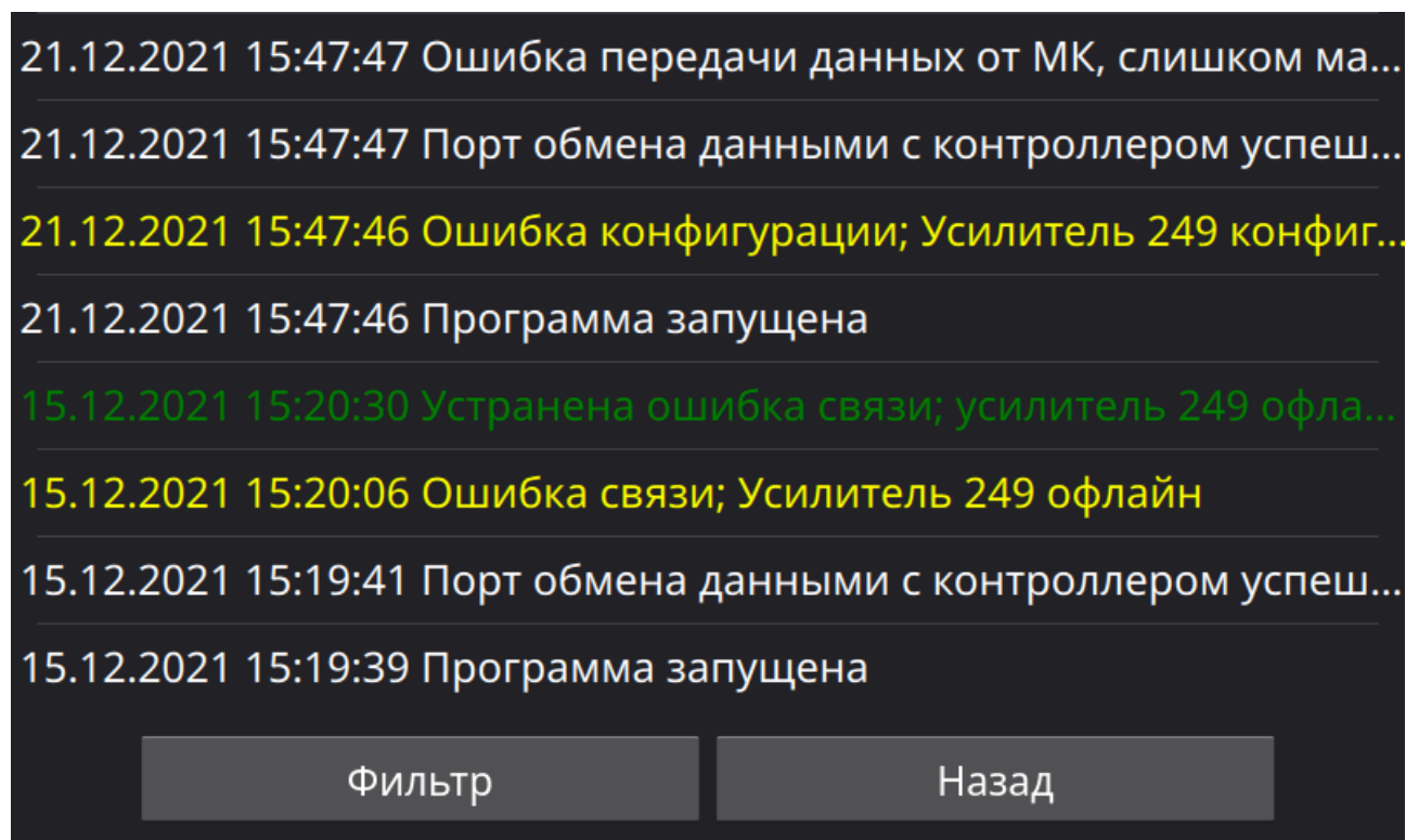
Рисунок 35 - Раздел «Журнал»
