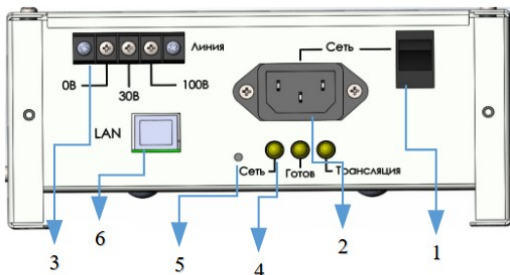
Рисунок 2 - Коммутационный отсек, вид снизу
