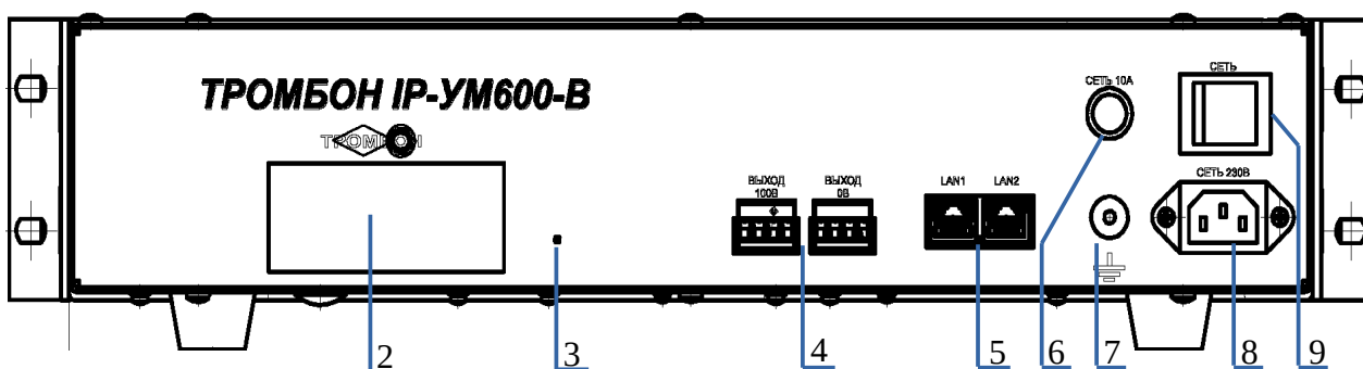
Рисунок 4 - Коммутационный отсек, вид сзади
